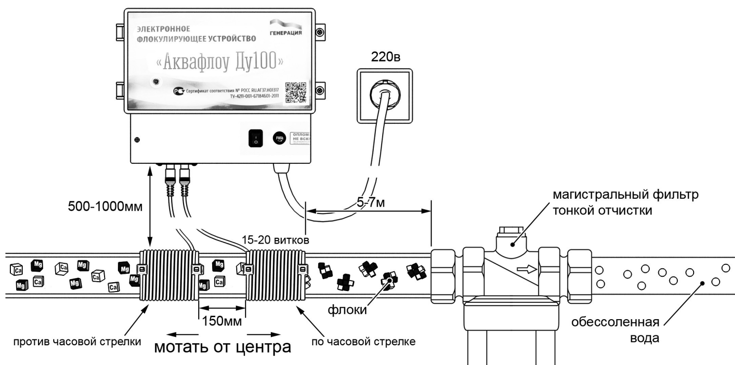
Рисунок 1. Условная схема монтажа прибора и магистрального фильтра
